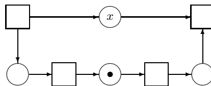
Fig. 1. Pr(x)
