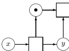
Fig. 5. Irp(x, y)
