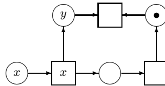
Fig. 3. Rpp(x, y)
